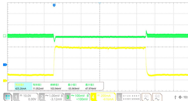
(17) Enable Start Up (VEN=12V, VOUT=3.3V, IOUT=0.6A)
